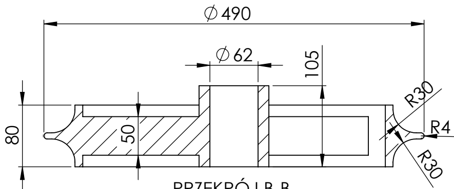
PRZEKRÓJ B-B SKALA 1 : 5
