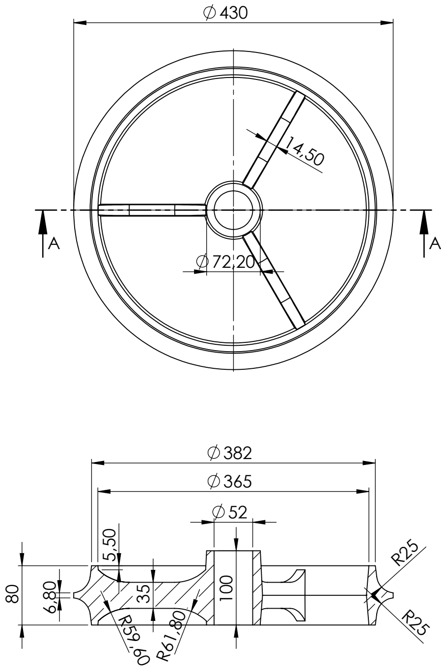
PRZEKRÓJ A-A SKALA 1 : 5
