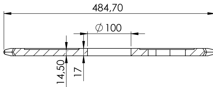
PRZEKRÓJ B-B SKALA 1 : 5
