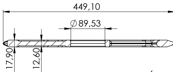
PRZEKRÓJ A-A SKALA 1 : 5
